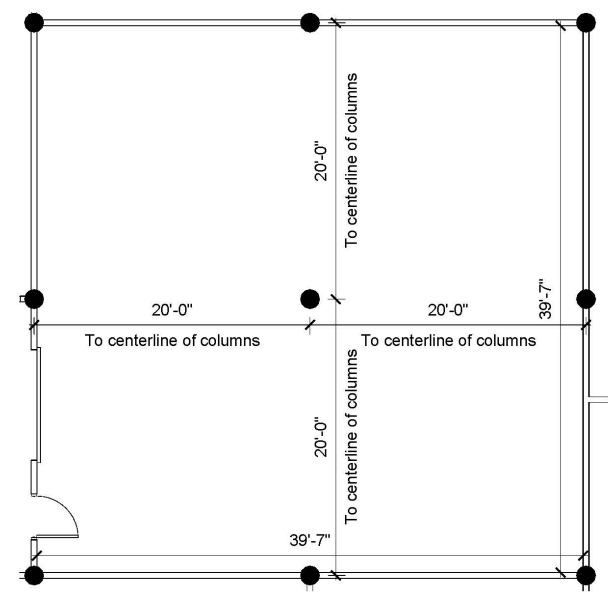
1 SUITE 105 N.T.S.
